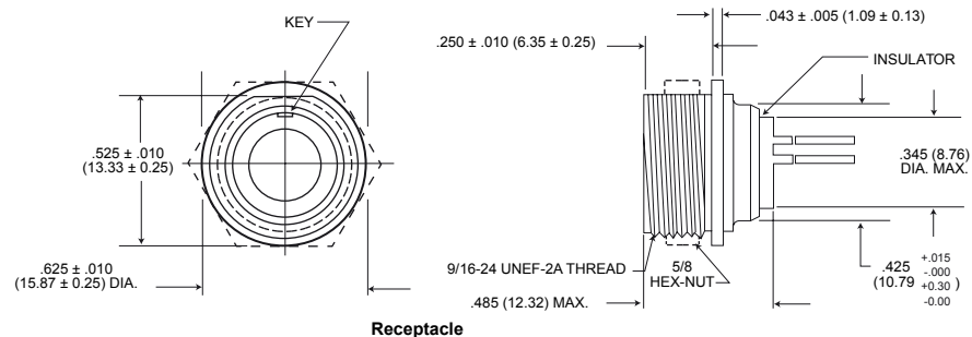
Receptacle
