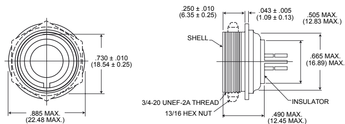
Receptacle
