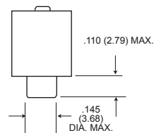
Receptacle
